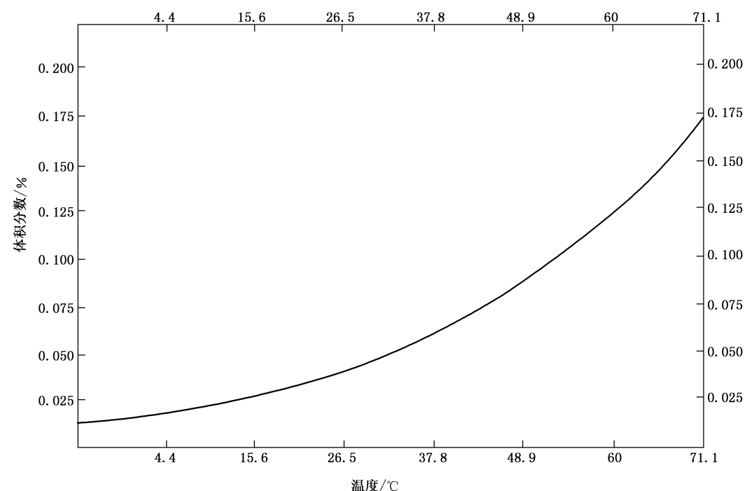
图 A.1 水在甲苯中的溶解度
